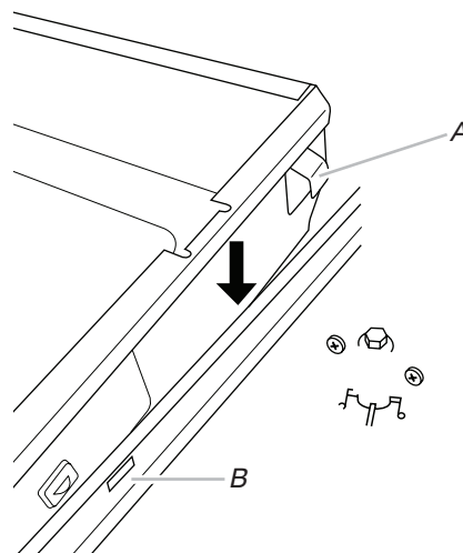
A. Onglet d'alignement du tiroir B. Encoche de glissière du tiroir
